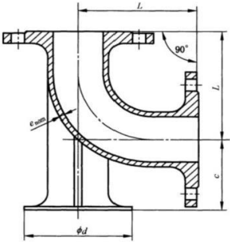
图 C.18 双盘 90° (1/4) 鸭掌弯头结构示意图
