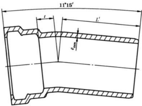
图 C.11 承插 11° 15′（1/32）弯头结构示意图
