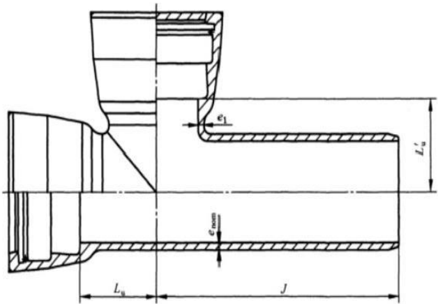
图 C. 15 承插单支承三通结构示意图
