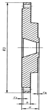
图 C. 27 PN25、PN40 减径法兰结构示意图
