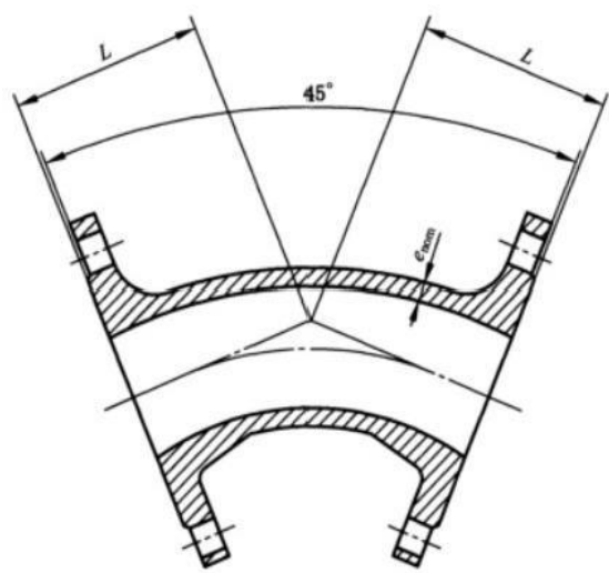
图 C.19 双盘 45°（1/8）弯头结构示意图
