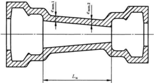
图 C. 16 双承减渐管结构示意图
