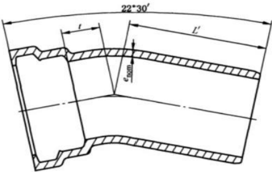
图 C. 10 承插 22° 30′（1/16）弯头结构示意图
