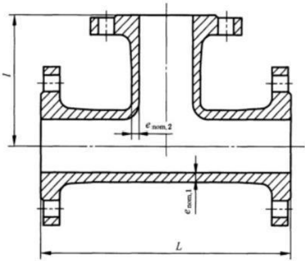
图 C. 20 全盘三通结构示意图
