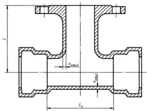
图 C.13 双承单支盘三通结构示意图
