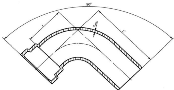
C.8 承插 90°（1/4）弯头结构示意图
