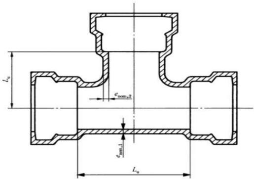
图 C.12 全承三通结构示意图
