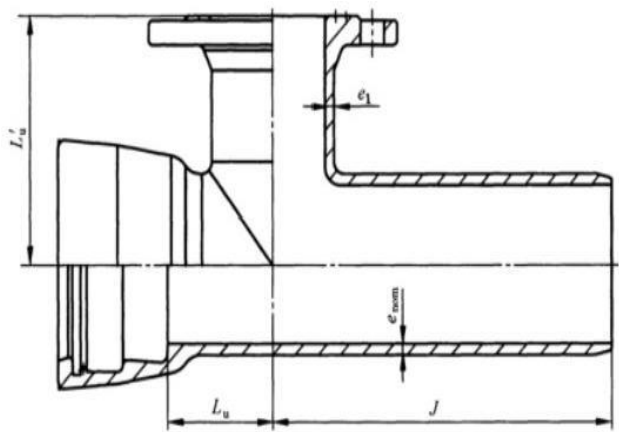
图 C. 14 承插单支盘三通结构示意图
