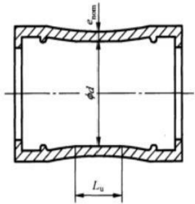
图 C.3 承套结构示意图
