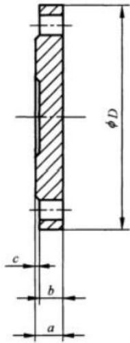
图 C.22 PN10 法兰盲板结构示意图
