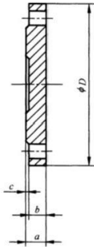
图 C.23 PN16 法兰盲板结构示意图
