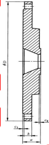
图 C. 26 PN10、PN16 减径法兰结构示意图
