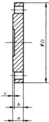
图 C. 24 PN25 法兰盲板结构示意图
