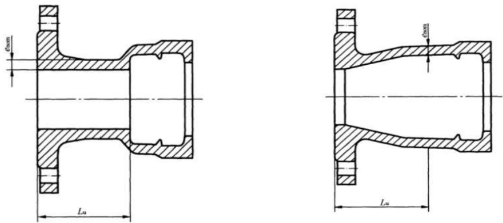
图 C.1 盘承结构示意图
