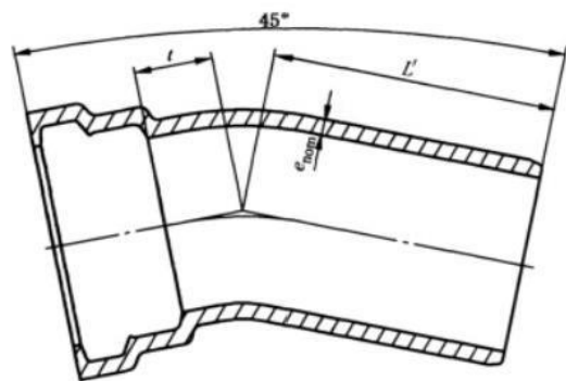
图 C.9 承插 45°（1/8）弯头结构示意图
