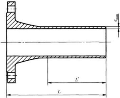
图 C.2 盘插结构示意图
