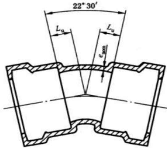
图 C.6 双承 22^{\circ}30' (1/16) 弯头结构示意图
