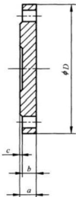
图 C. 25 PN40 法兰盲板结构示意图
