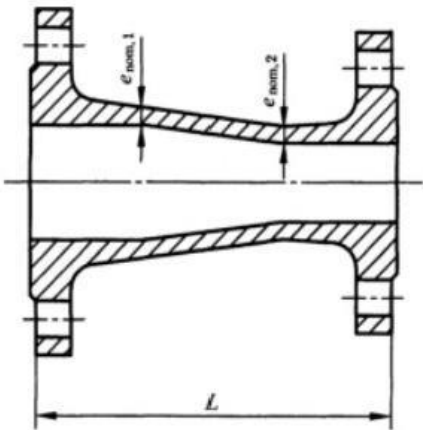
图 C.21 双盘渐缩管结构示意图
