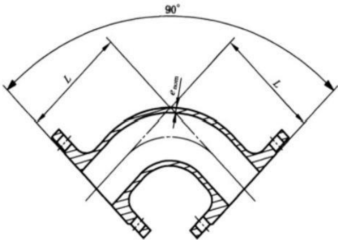
图 C.17 双盘 90°（1/4）弯头结构示意图
