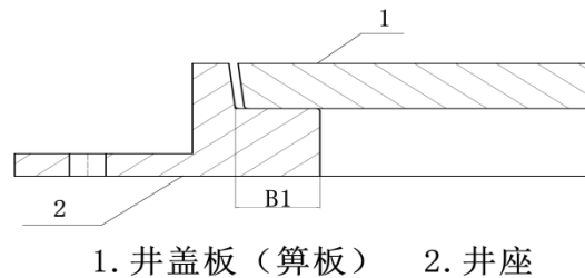
图 2 井座上与井盖板或算板接触部位的宽度
