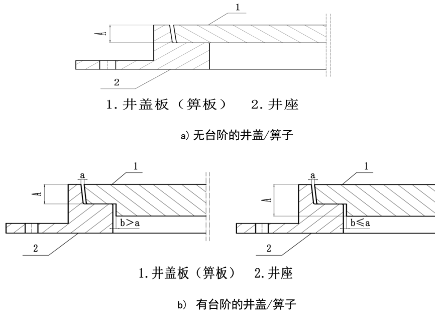
图 1 嵌入深度
